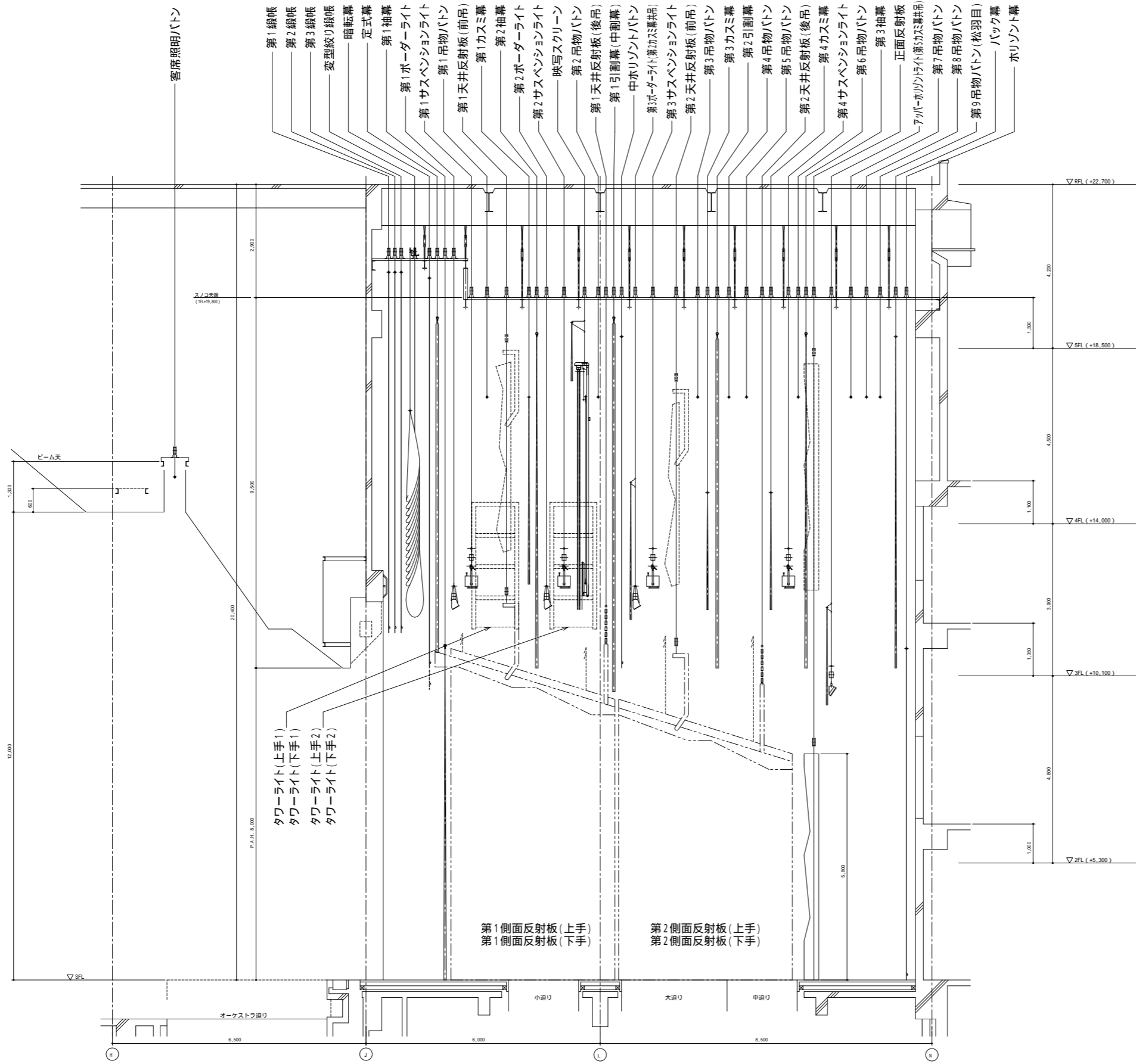
板橋区立文化会館 / 大ホール / 舞台断面図 / S = 1 / 100
