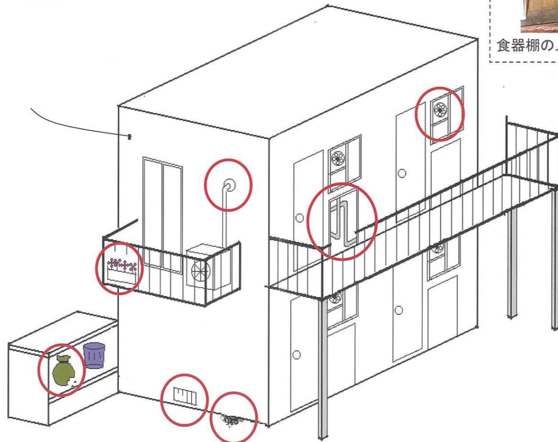
メーターボックス内の配管貫通部
