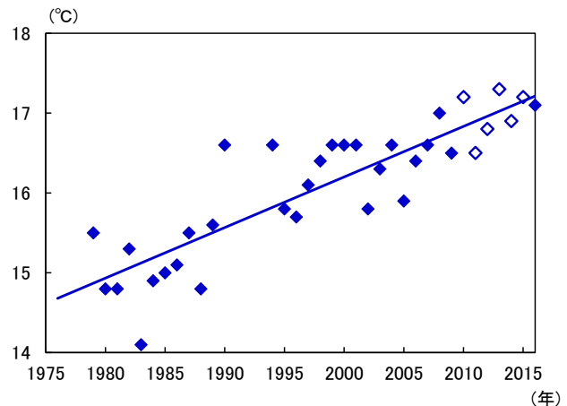
図2-1-4 板橋区（氷川町※）の平均気温の推移
