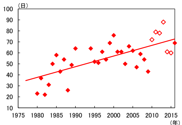
図2-1-6 板橋区（氷川町※）の最高気温が30℃以上（真夏日）の日数の推移
