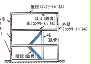
例) 鉄骨造の準耐火建築物
