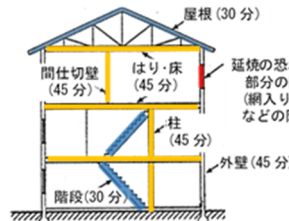
例) 木造の準耐火建築物
