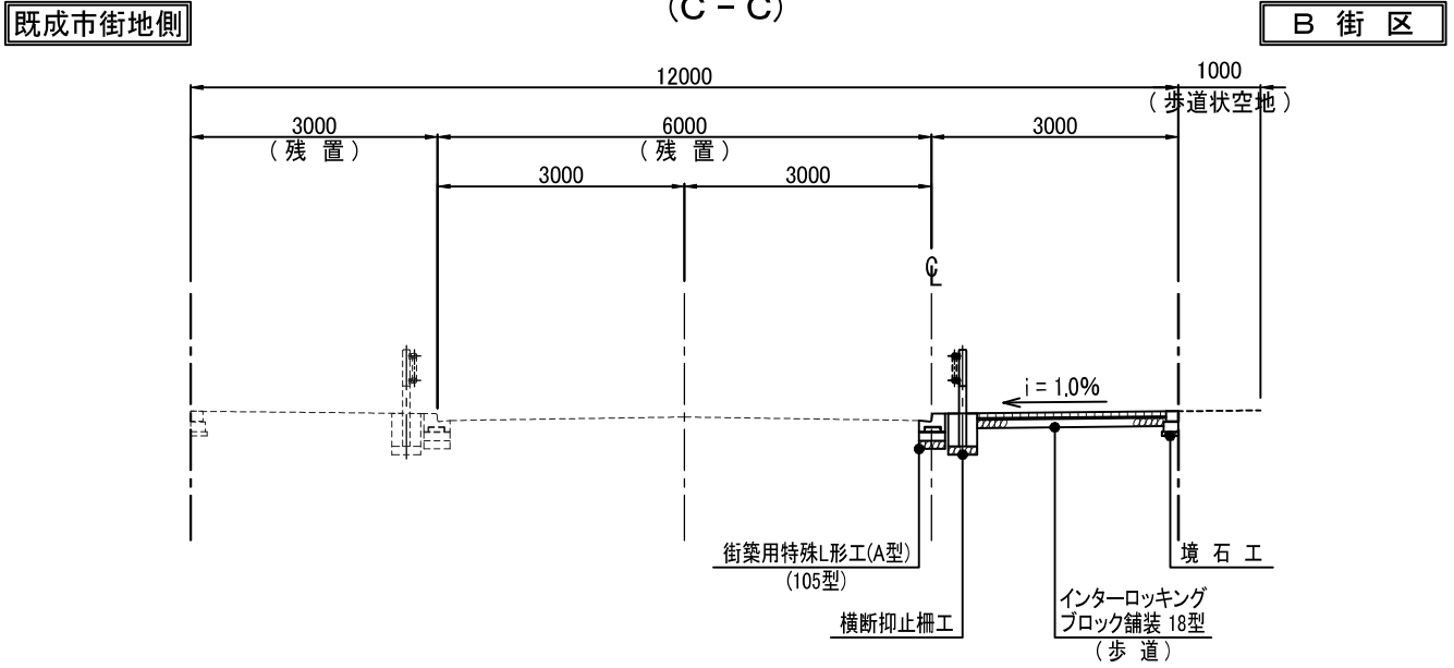
板橋特別区道第2091号線 (都市計画道路駅街路第1号線) (C - C)
