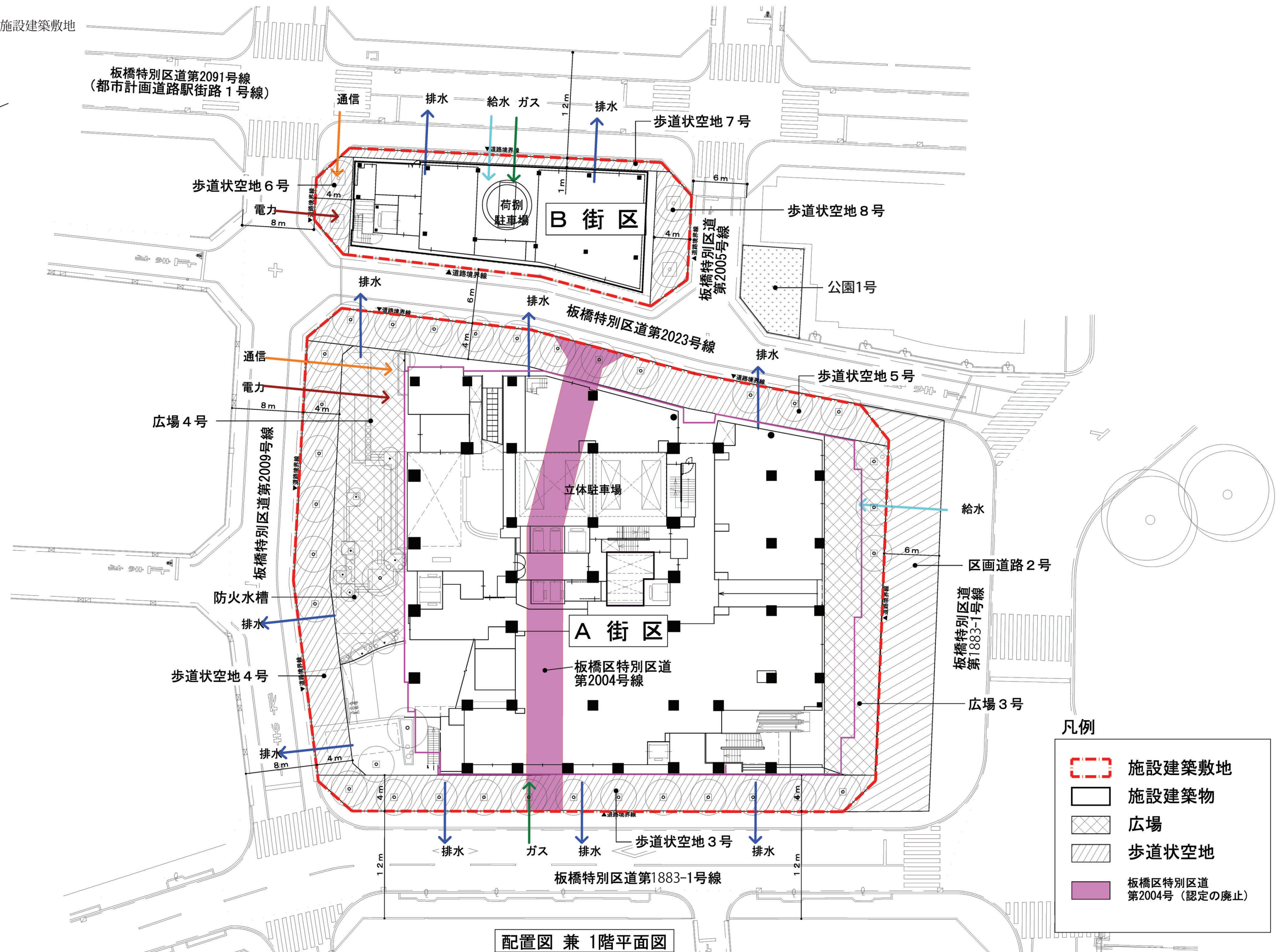
配置図兼1階平面図 S=1:400(A3)
