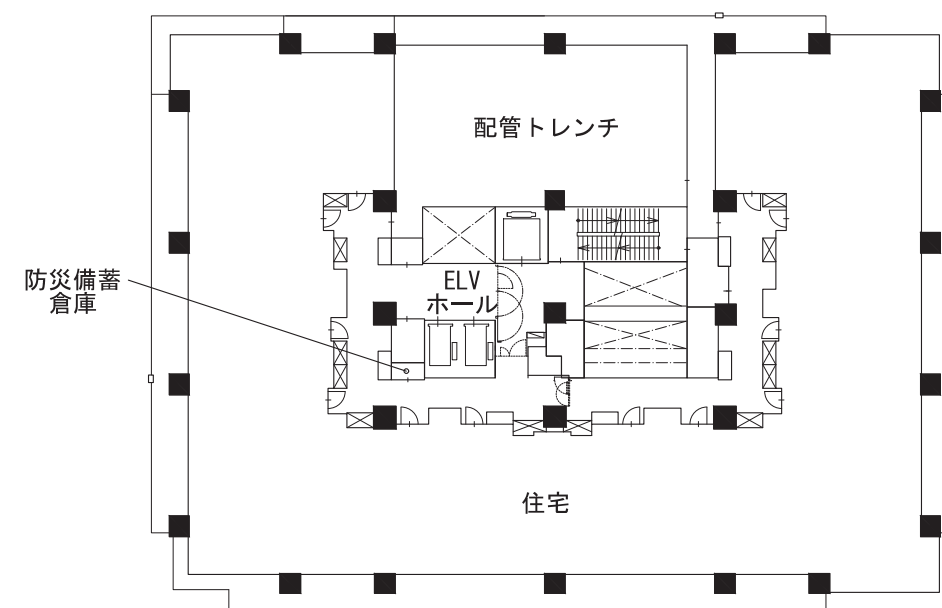
16階平面図
