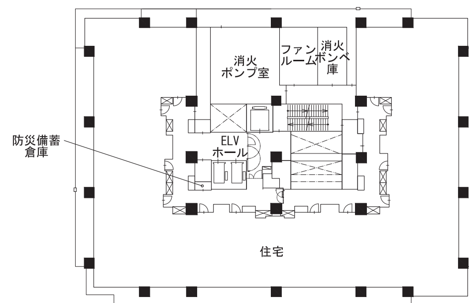
15階平面図
