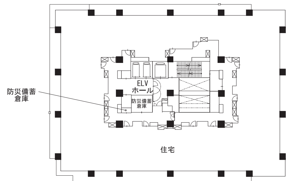
19階-22階平面図
