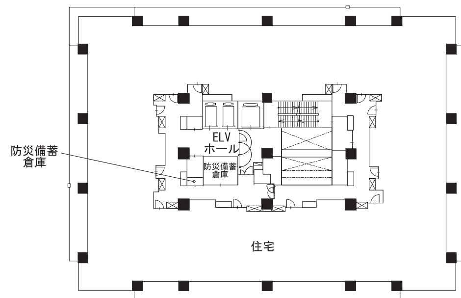
36階-37階平面図
