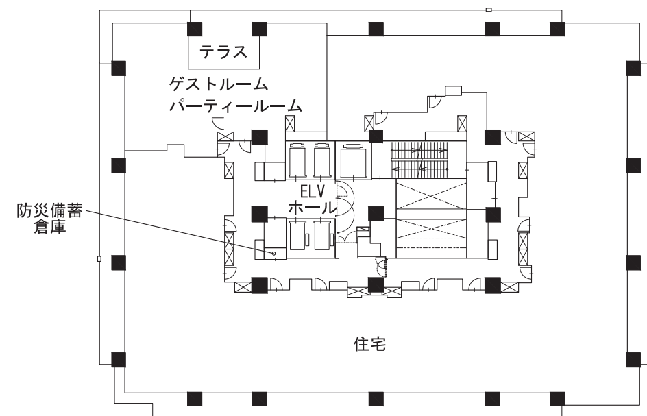
17階平面図
