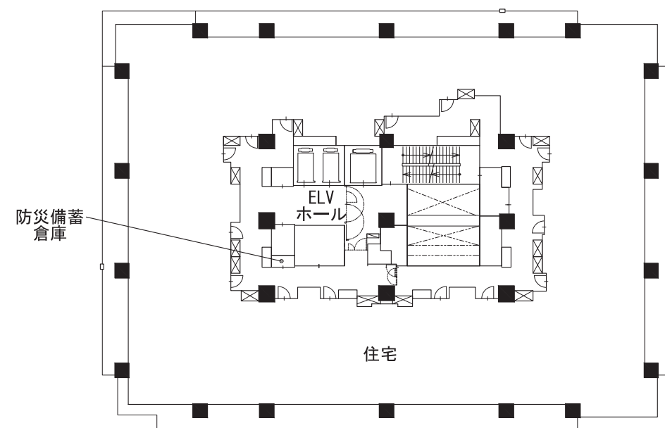
18階平面図
