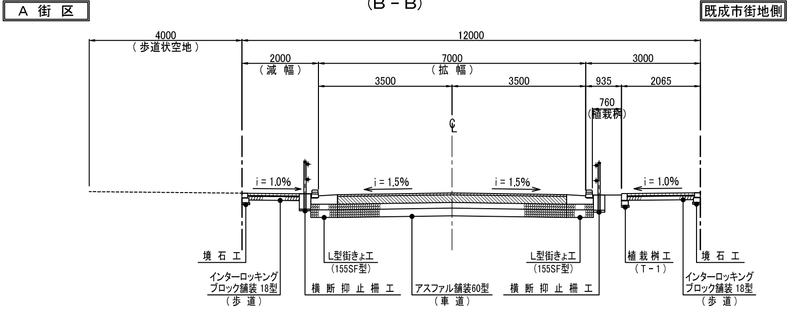
(一 般 部) 板橋特別区道第1883-01号線 (B - B)
