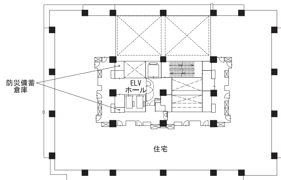
14階平面図
