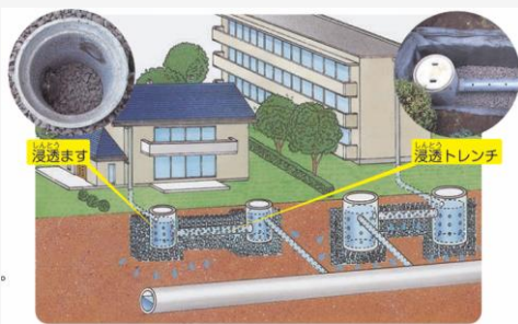
図表：浸透施設のイメージ 出典：東京都総合治水対策協議会パンフレット
