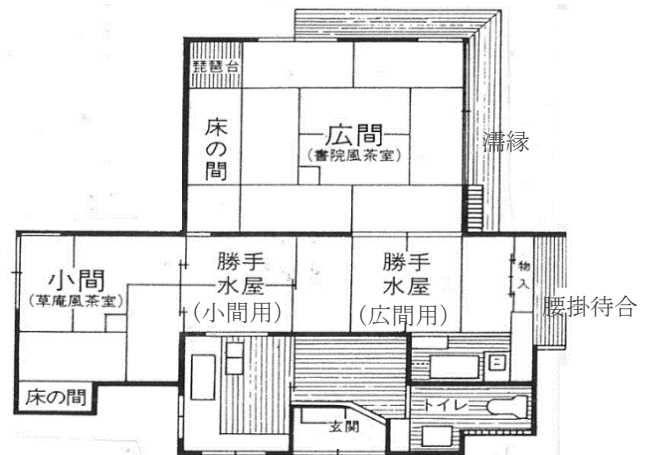
茶室平面図
