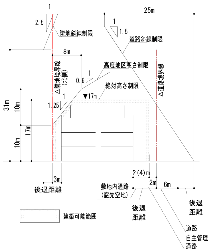
図V-4 高さ制限の検討図
