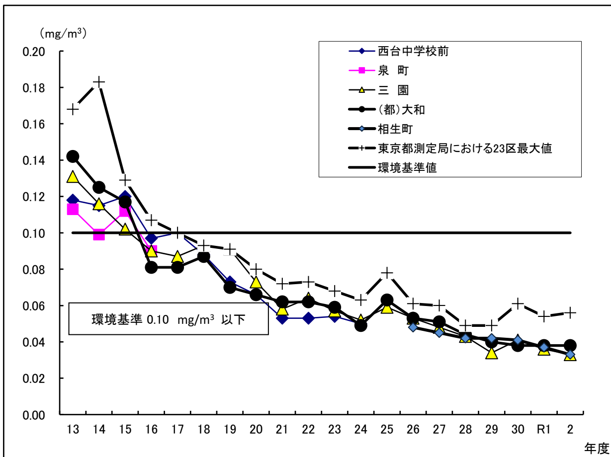
日平均値の2%除外値(道路沿道測定室)の経年変化グラフ
