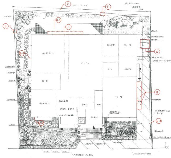
配置図 S=1:200
