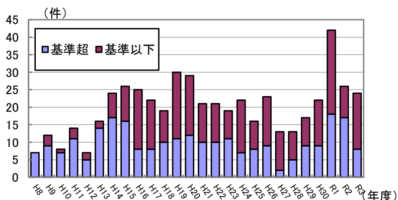
図2-4-9 土壤汚染調査実績
