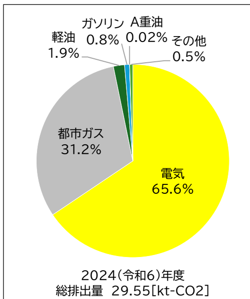
図1 エネルギー別の排出割合
