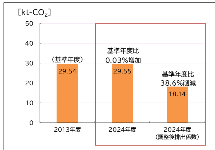
図2 温室効果ガス総排出量
