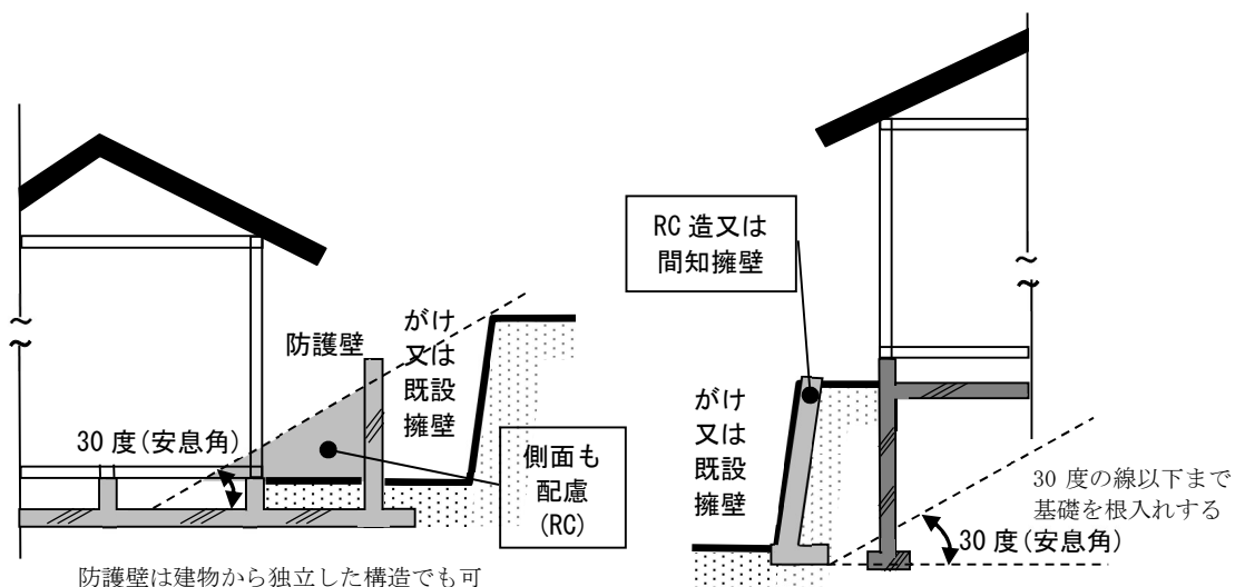
① がけの下に敷地に建築する場合の例 防護壁を設ける場合
