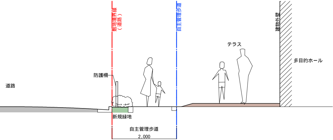
A断面
