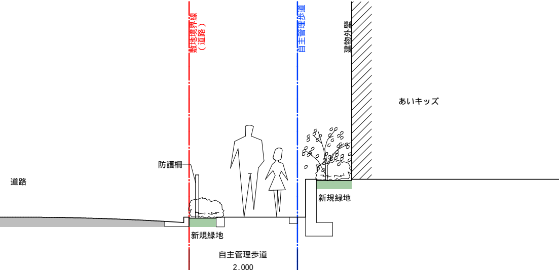
E断面
