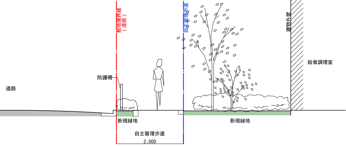
B断面
