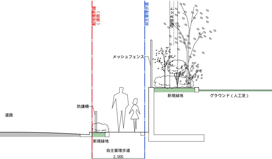
D断面
