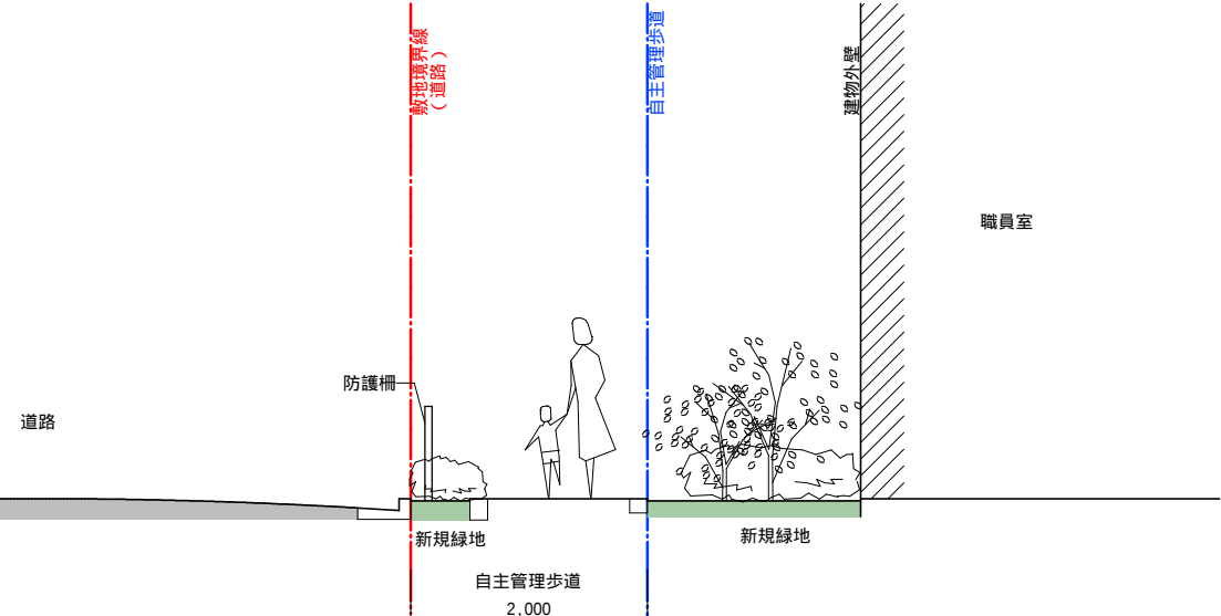
C断面
