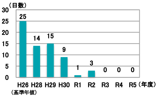
図2-4-1 PM2.5の基準値Bレベル以上（35 μg/m³超）の日数
