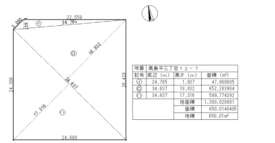
求積図
