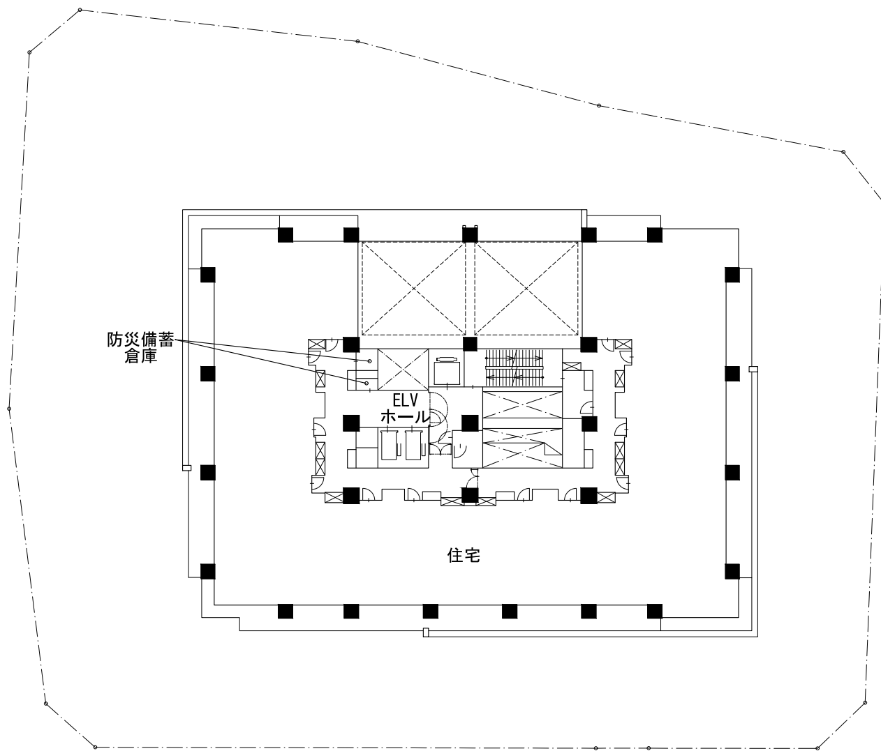
6階-14階平面図
