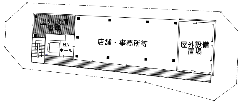
B地区 6階平面図
