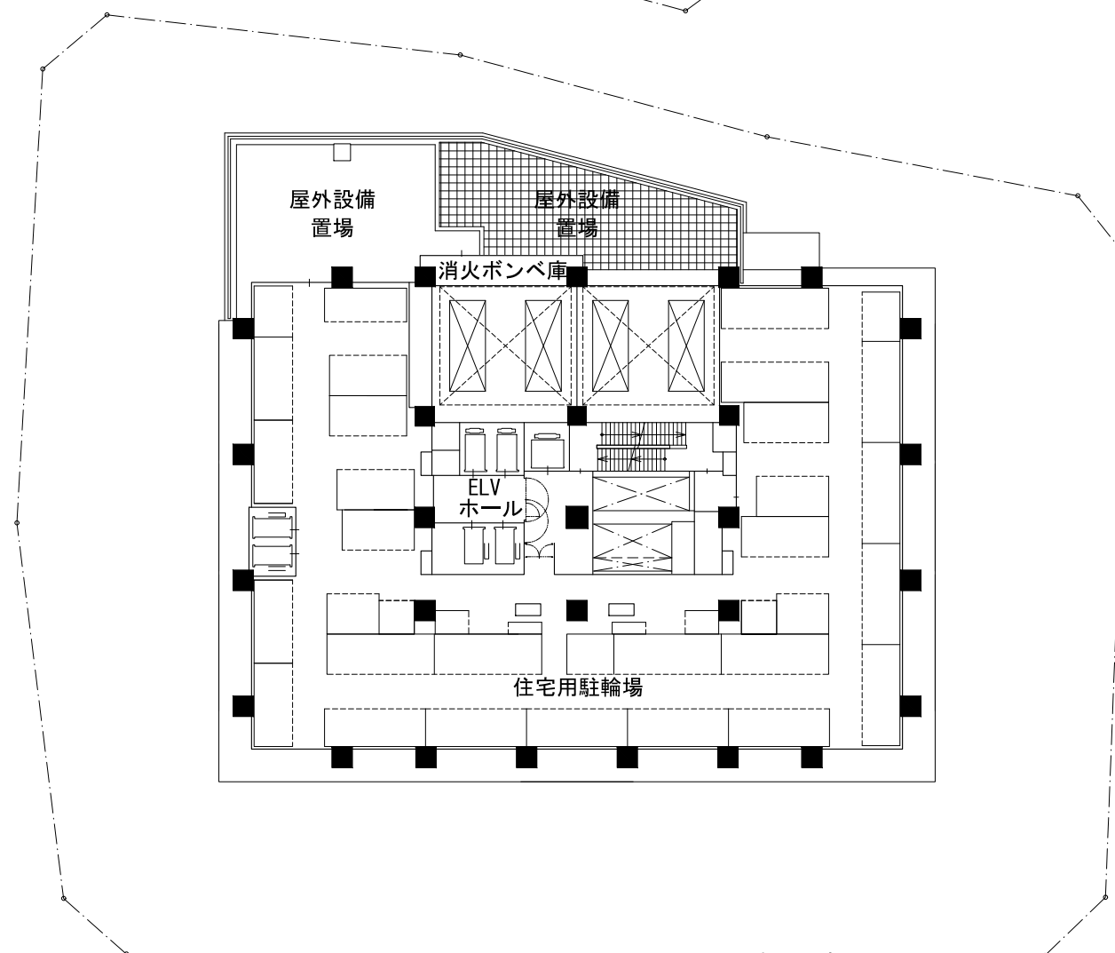
B地区 5階平面図
