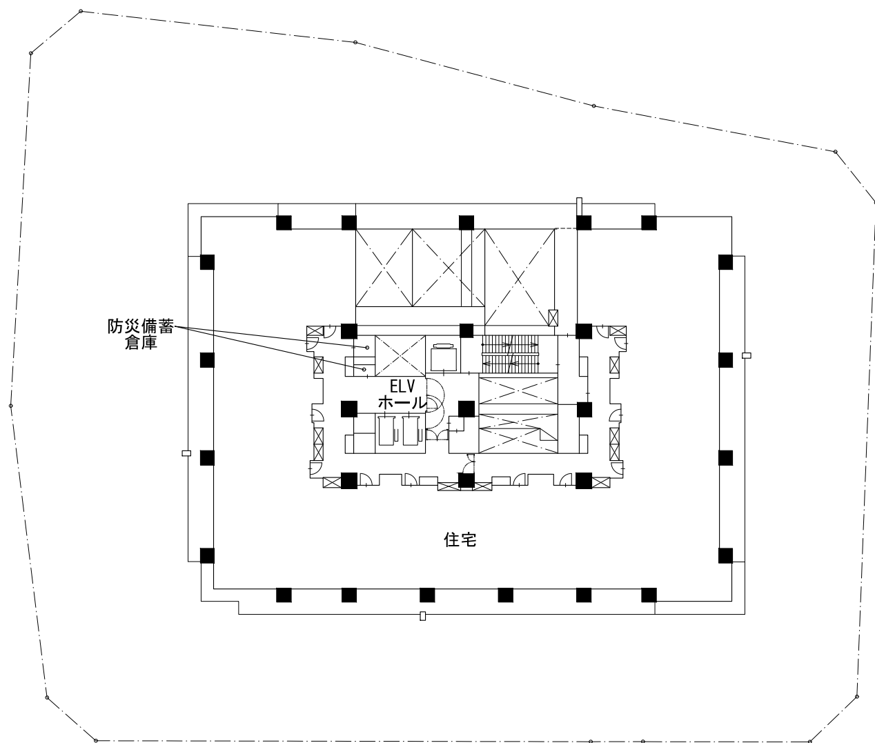
16階平面図
