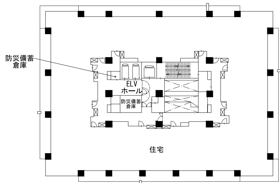
23階-35階平面図
