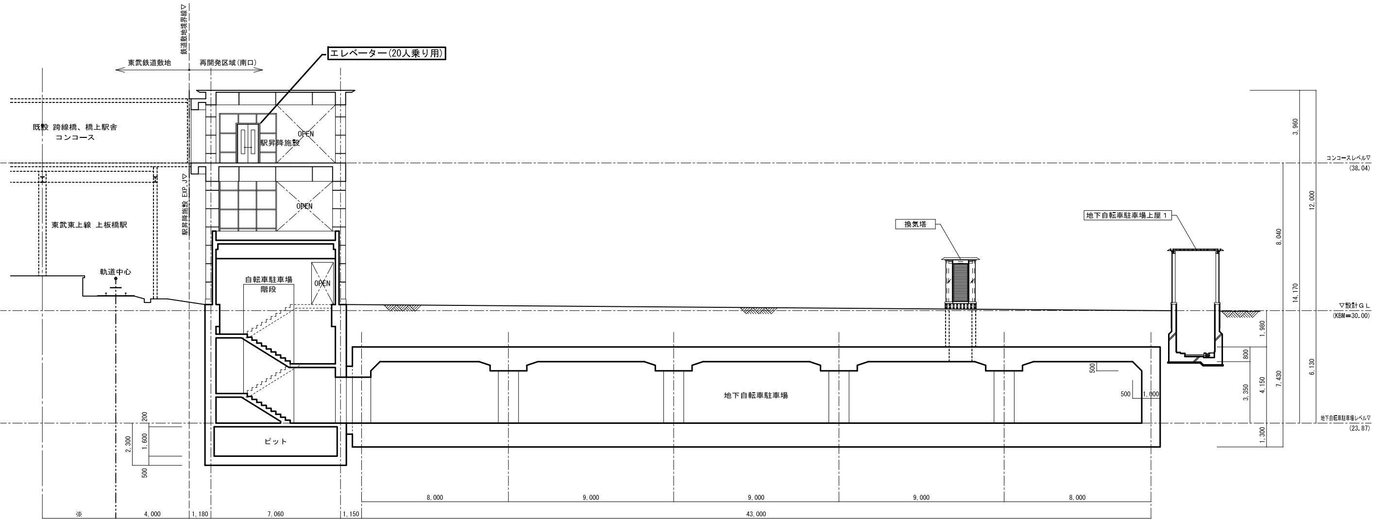
A-A 断面図 1:200
