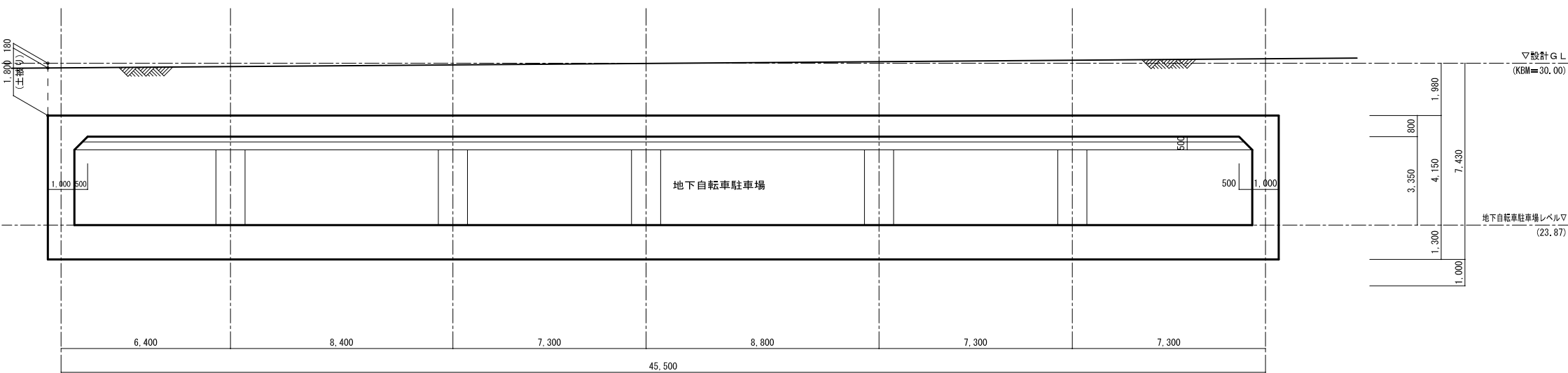
B-B 断面図 1:200
