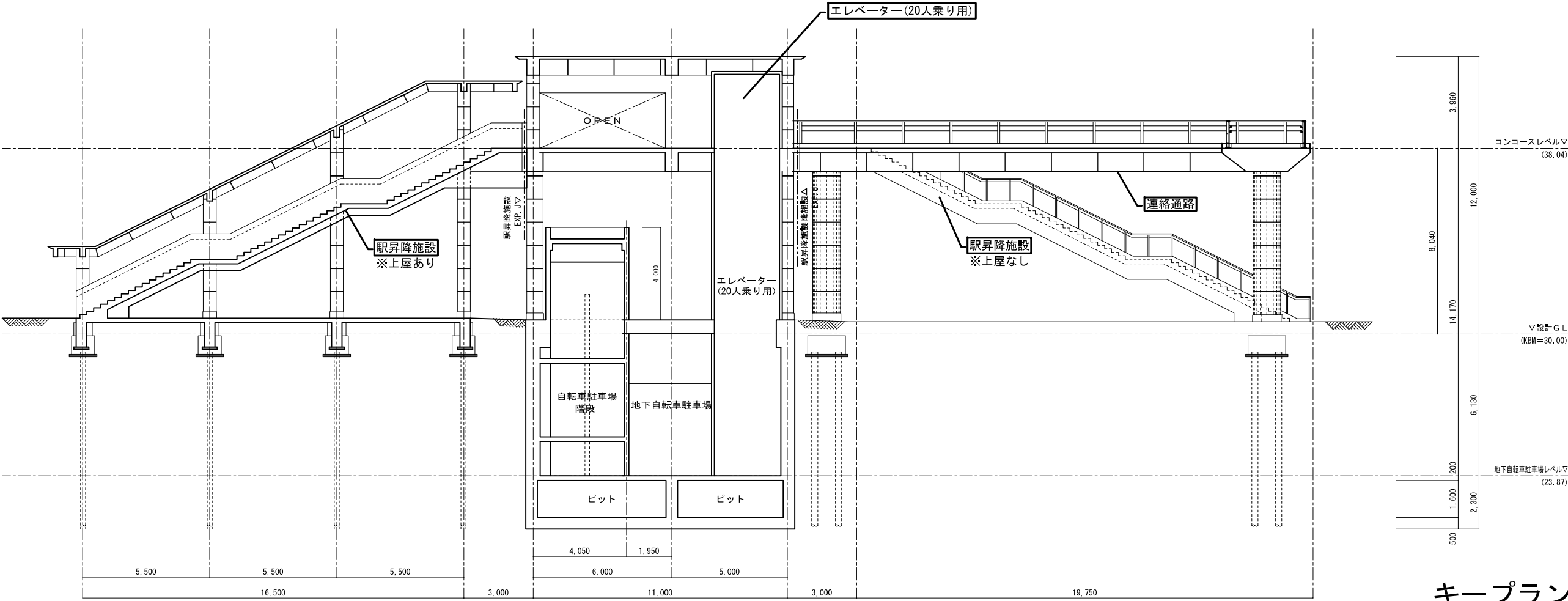
C-C 断面図 1:200
