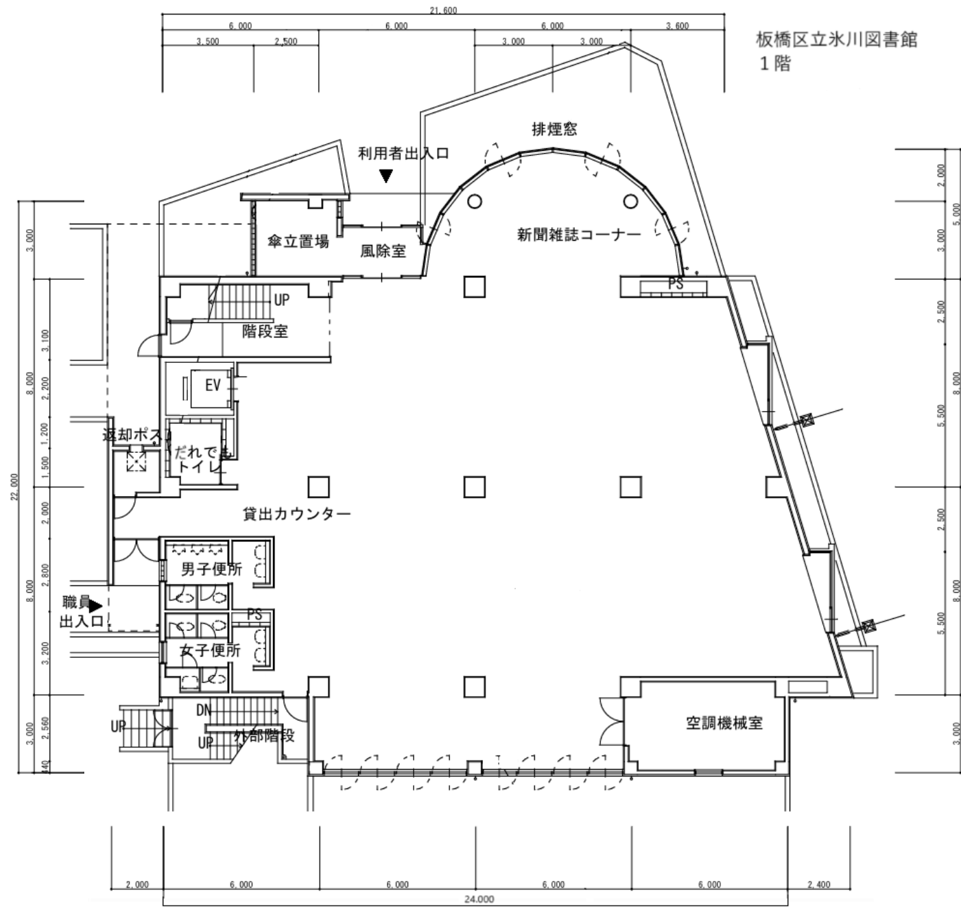
板橋区立氷川図書館 1階・2階 平面図
